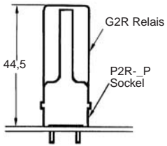
G2R-□P
