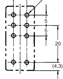
Befestigungsbohrungen
