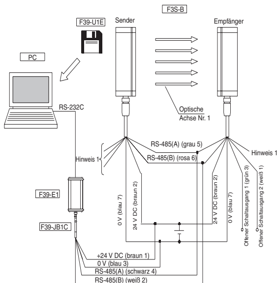
Hinweis 1: Informationen zur Verkabelung des Sicherheitslichtgitters F3S-B finden Sie in der Bedienungsanleitung des Sicherheitslichtgitters.
